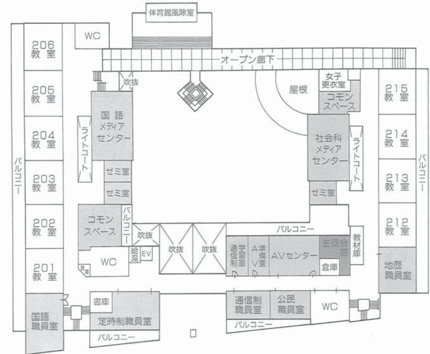
2階平面図
