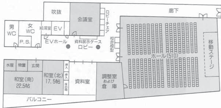
玉翠会館平面図
